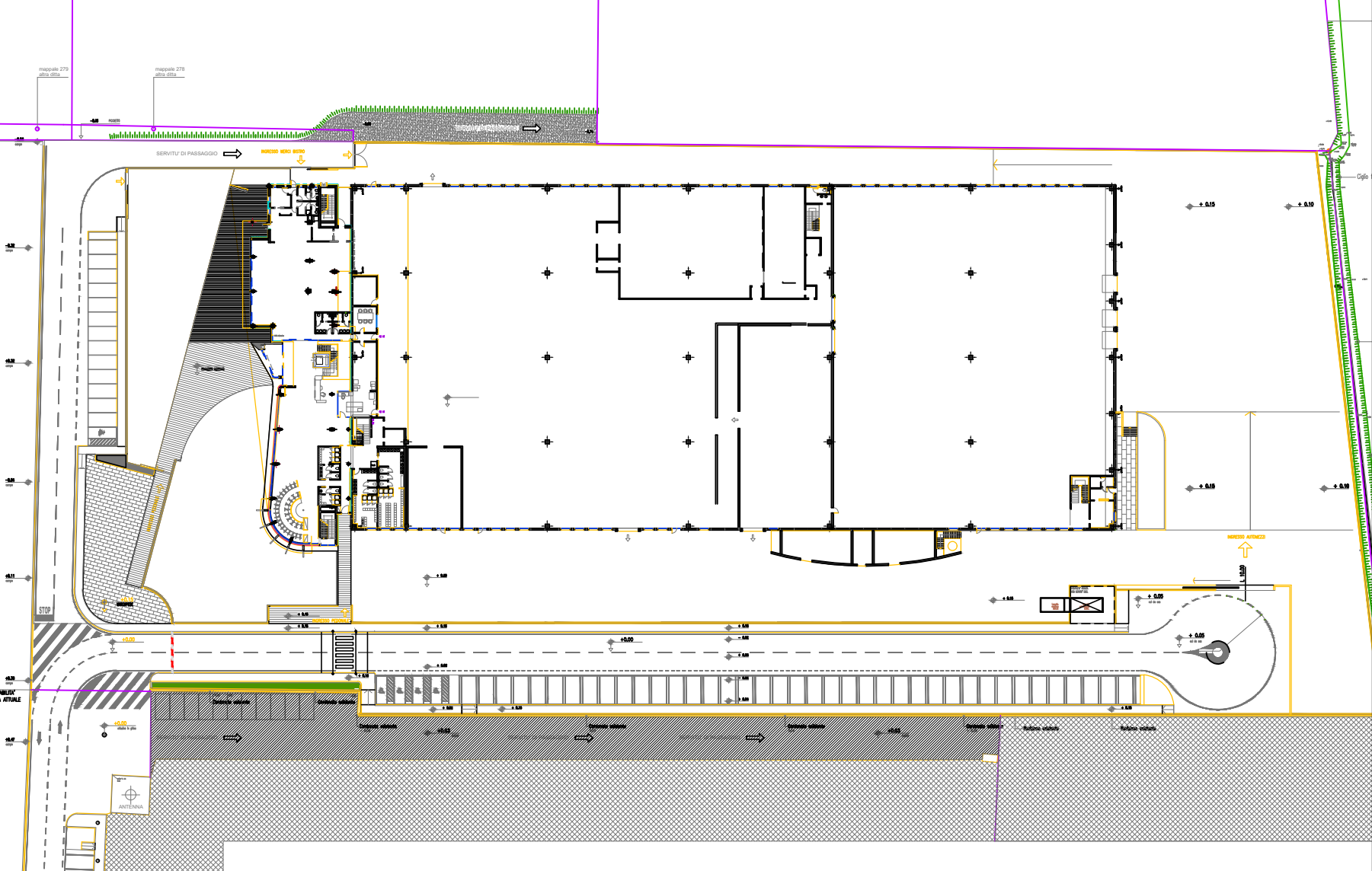
Planimetria - scala 1:1000
